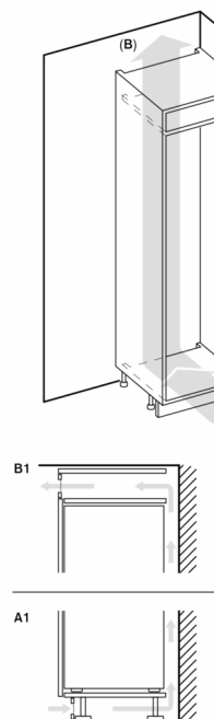
A: Entrée d'air \geq 200 \text{ cm}^2 ; options d' B: Sortie d'air \geq 200 \text{ cm}^2 ; options de
